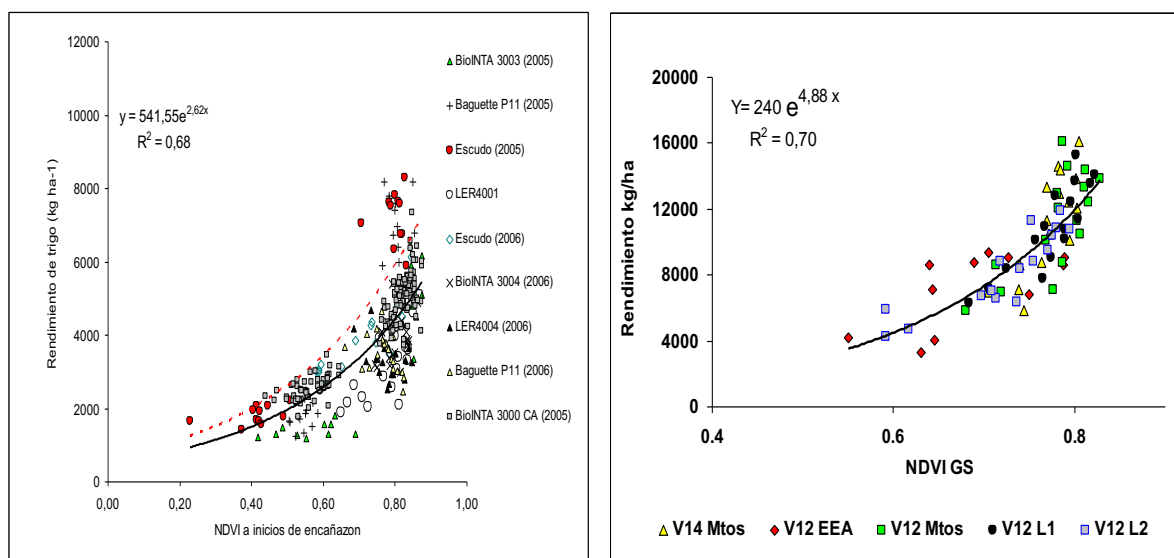
Figura 6. Predicción del rendimiento para trigo (izquierda) y maíz (derecha) en Paraná (Argentina) a partir del índice normalizado de diferencias de vegetación (NDVI) utilizando sensores remotos. Adaptado de Melchiori (2012).
