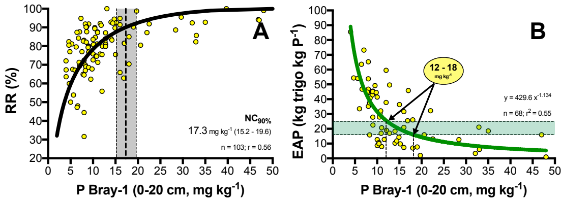
Figura 3. Estimación de nivel crítico de P extractable Bray-1 utilizando rendimiento relativo (RR, A) y eficiencia agronómica de la respuesta a P (EAP, B). En A, la franja vertical gris indica el intervalo de confianza (95%) para el nivel crítico. Para lograr el 90% de RR es necesario tener entre 15.2 y 19.6 \text{mg kg}^{-1} . En B, la franja horizontal verde indica el percentil central (P25-P75) de la relación histórica de precios de P en trigo (16 a 25 \text{kg trigo kg P}^{-1} ). Según la función ajustada y la relación de precios, el umbral de P Bray-1 que determina respuestas económicas varía entre 12 y 18 \text{mg kg}^{-1} . Datos correspondientes a 103 ensayos de fertilización fosfatada en la región pampeana (1998-2014) de distintos autores. Fuente: Correndo y García (2016).
