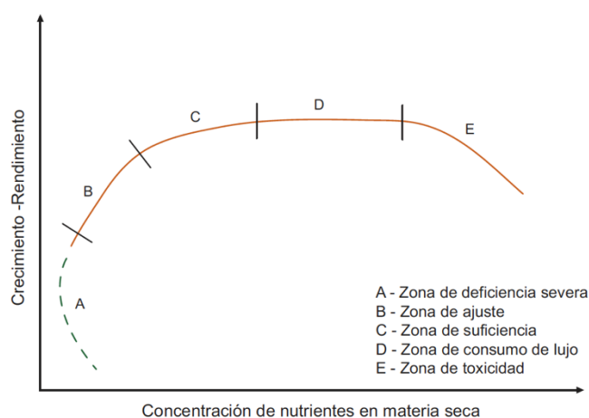
Figura 4. Relación general entre el crecimiento y/o rendimiento y el contenido de nutrientes en tejido vegetal. Adaptado de Jones (1998).
