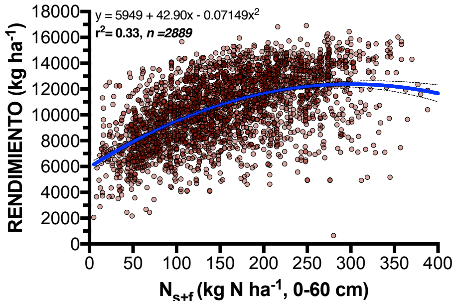
Figura 2. Rendimiento de maíz en función de la disponibilidad de N (como N en el suelo -0-60cm- a la siembra del cultivo + N de fertilizante). Datos de 545 ensayos distribuidos en la región pampeana (Buenos Aires, Santa Fe, Córdoba, Entre Ríos, La Pampa y San Luis) en el período 1994-2014. Regresión significativa ( p < 0.0001 ). Adaptado de Correndo (2016).
