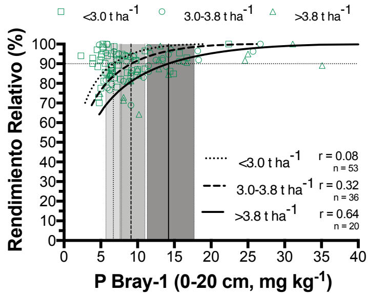
Figura 3.14. Relación entre RR y el nivel de P Bray-1 (0-20 cm) para soja en Argentina segregando sub-sets de datos por cultivo según potencial de rendimiento y clase textural. Argentina. Campañas 1971/72 a 2016/17. Las franjas verticales grises indican el nivel crítico con su respectivo intervalo de confianza (95%).
