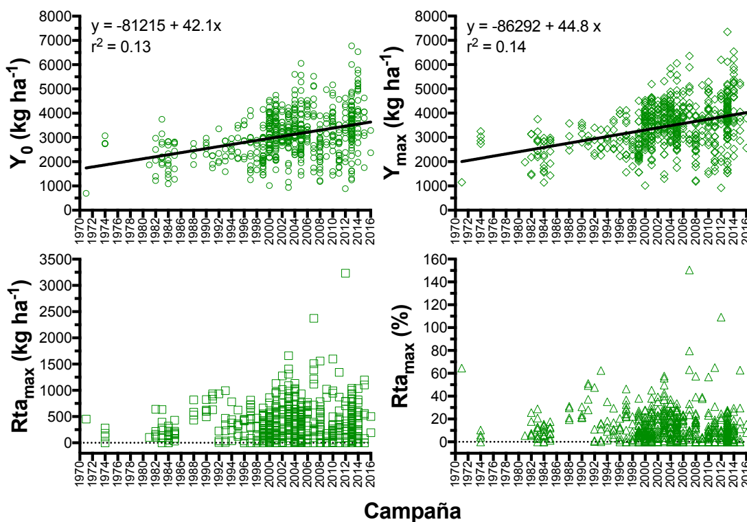
Figura 3.6. Evolución temporal del rendimiento de soja sin P ( Y_0 ), rendimiento máximo observado ( Y_{max} ), y respuesta máxima ( Rta_{max} ) absoluta y porcentual en los ensayos de la base de datos ( n=377 ). Argentina. Campañas 1971/72 a 2016/17.
