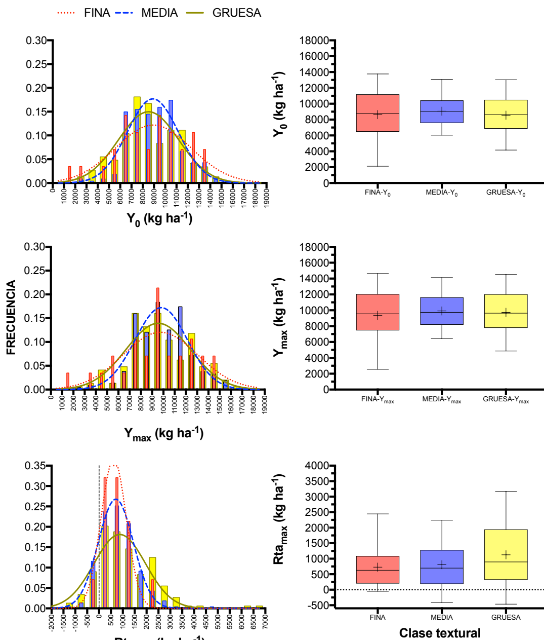
Figura 3.7. Distribución empírica (izquierda) y diagramas boxplot (derecha) de niveles de rendimiento testigo ( Y_0 ), rendimiento máximo ( Y_{max} ) y respuesta máxima observada ( Rta_{max} ) en los ensayos de fertilización con P en maíz según clase textural del suelo. Argentina. Campañas 1980/81 a 2015/16. En los boxplot: las barras verticales indican percentiles 5% y 95%, las cajas los percentiles 25% y 75%, la línea horizontal la mediana o percentil 50%, y los signos “+” indican la media.
