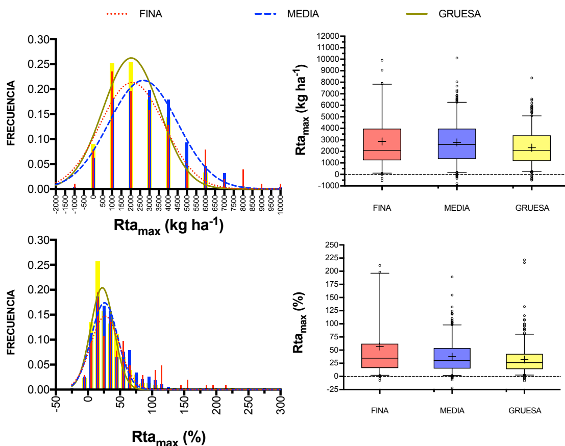
Figura 4.7. Distribución empírica y frecuencia acumulada de potencial de respuesta a N ( Rta_{max} ) en términos absolutos (kg ha -1 ) y relativos (%) en los ensayos de fertilización con N en maíz para tres clases texturales de suelo. Argentina. Campañas 1980/81 y 2016/17. En los boxplot: las barras verticales indican percentiles 5% y 95%, las cajas los percentiles 25% y 75%, la línea horizontal la mediana o percentil 50%, y los signos “+” indican la media.
