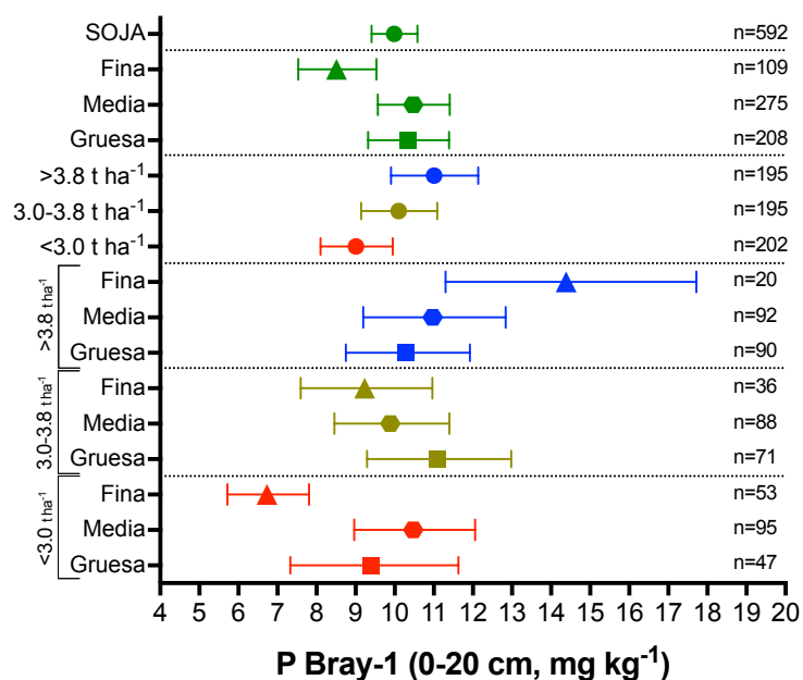
Figura 3.17. Comparación de niveles críticos de P-Bray-1 (0-20 cm) estimados para el logro del 90% del rendimiento relativo en el cultivo de soja ( AS_{C90\%} ), utilizando el set de datos completo (todos) o segregado según potencial de rendimiento, clase textural del suelo, y la interacción potencial de rendimiento x clase textural. Las barras horizontales indican el intervalo de confianza de los niveles críticos (95%). Superposición significa ausencia de diferencias significativas.
