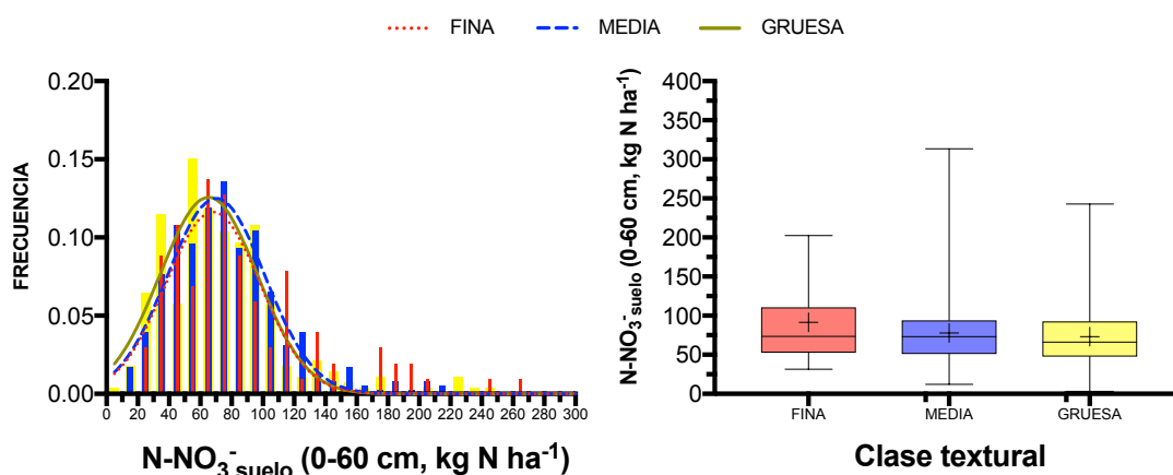
Figura 4.3. Distribución empírica (izquierda) y diagrama boxplot (derecha) de niveles de N-NO_3^- (0-60cm) según clase textural de suelo para los ensayos de fertilización con N en maíz. En el boxplot, las barras verticales indican los percentiles 5% y 95%, las cajas los percentiles 25% y 75%, la línea horizontal la mediana, y el signo “+” indica la media.
