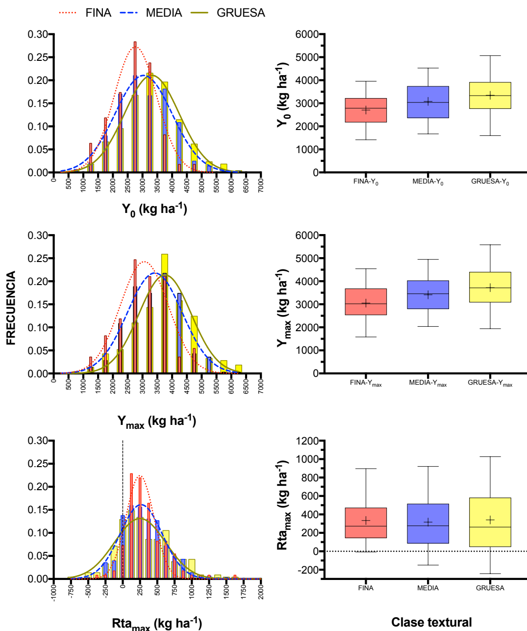
Figura 3.8. Distribución empírica (izquierda) y diagramas boxplot (derecha) de niveles de rendimiento testigo ( Y_0 ), rendimiento máximo ( Y_{max} ) y respuesta máxima observada ( Rta_{max} ) en los ensayos de fertilización con P en soja. Argentina. Campañas 1971/72 a 2016/17. En los boxplot: las barras verticales indican percentiles 5% y 95%, las cajas los percentiles 25% y 75%, la línea horizontal la mediana o percentil 50%, y los signos “+” indican la media.
