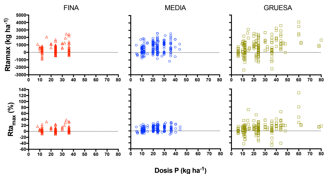
Figura Anexo 2. Variación de la respuesta a P en maíz ( Rta_{max} ) en términos absolutos ( kg ha^{-1} ) y relativos (%) para las tres clases texturales de suelo en función de la dosis de P ( kg P ha^{-1} ) para los ensayos bajo estudio
