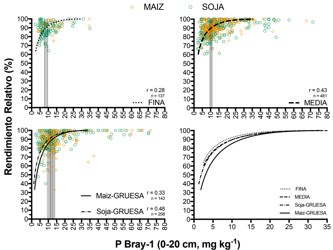
Figura 3.10. Relación entre RR y el nivel de P Bray-1 (0-20 cm) para maíz y soja en Argentina según 3 clases texturales de suelo. Las curvas indican el ajuste del modelo bivariado estimado mediante el método ALCC-modificado. Argentina. Campañas 1971/72 a 2016/17. Las franjas verticales grises indican el nivel crítico con su respectivo intervalo de confianza (95%).
