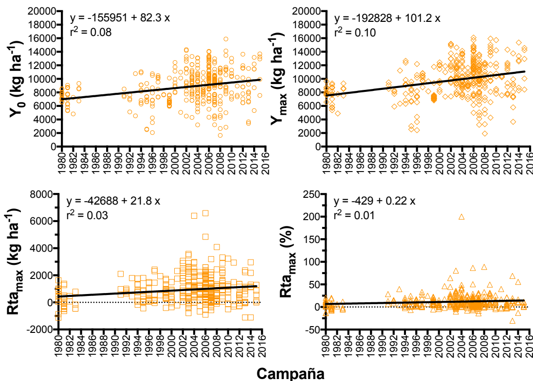
Figura 3.5. Evolución temporal del rendimiento de maíz sin P ( Y_0 ), rendimiento máximo observado ( Y_{\max} ), y respuesta máxima ( Rta_{\max} ) absoluta y porcentual en los ensayos de la base de datos ( n=377 ). Argentina. Campañas 1980/81 a 2015/16.
