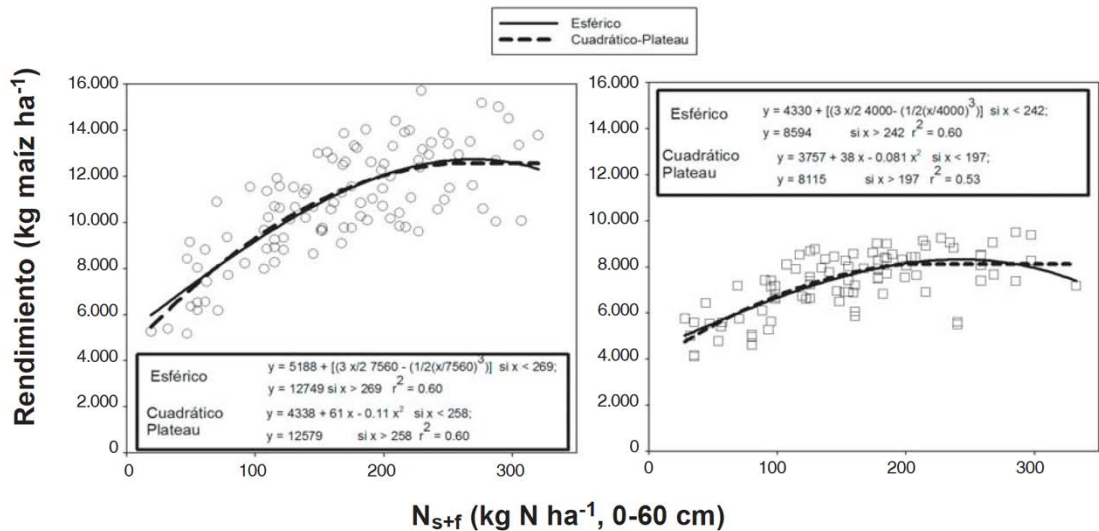
Figura 1.3. Rendimiento de maíz en función de la disponibilidad de N (como N en el suelo -0-60cm- a la siembra del cultivo + N de fertilizante) en ambientes de mayor (izquierda) y menor potencial de rendimiento (derecha) de la región pampeana norte (39 ensayos). Fuente: Salvagiotti et al. (2011).
