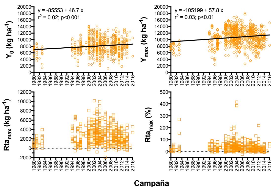
Figura 4.5. Evolución temporal del rendimiento de maíz sin N ( Y_0 ), rendimiento máximo observado ( Y_{\text{max}} ), y respuesta máxima ( Rta_{\text{max}} ) absoluta y porcentual en los ensayos de la base de datos ( n=788 ). Argentina. Campañas 1980/81 a 2016/17.
