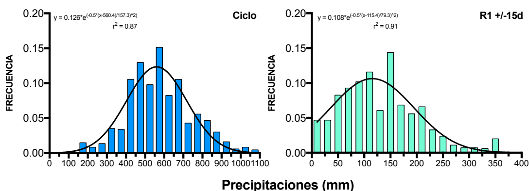
Figura 4.4. Distribución de las precipitaciones durante el ciclo y alrededor de floración, correspondiente a la base de datos de ensayos de fertilización nitrogenada en maíz (n=788). Argentina. Campañas 1980/81 a 2016/17.
