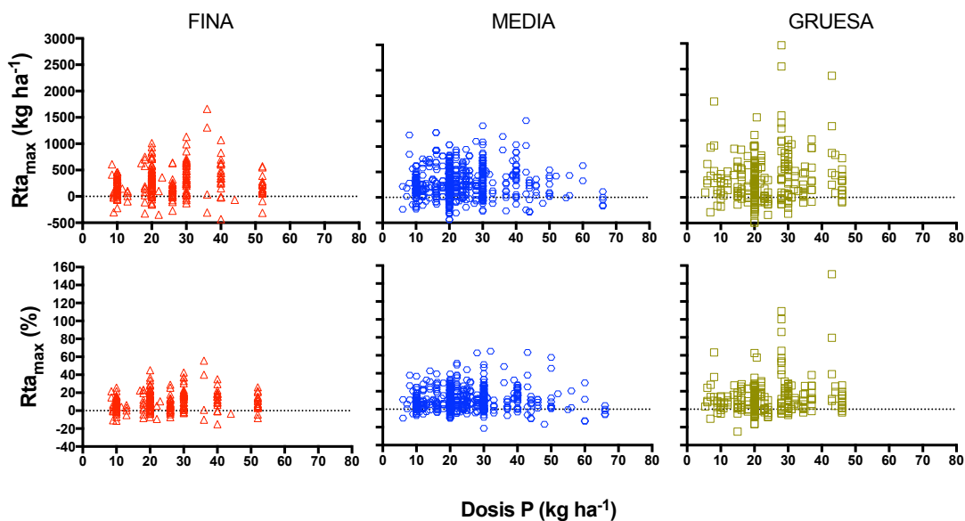
Figura Anexo 3. Variación de la respuesta a P en soja ( Rta_{max} ) en términos absolutos ( kg\ ha^{-1} ) y relativos (%) para las tres clases texturales de suelo en función de la dosis de P ( kg\ P\ ha^{-1} ) para los ensayos bajo estudio.
